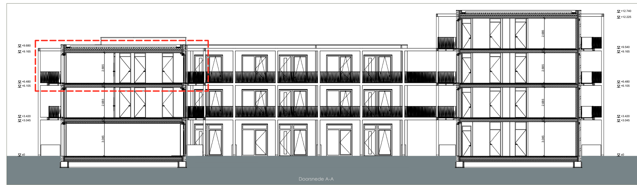
Doorsnede 1:200
