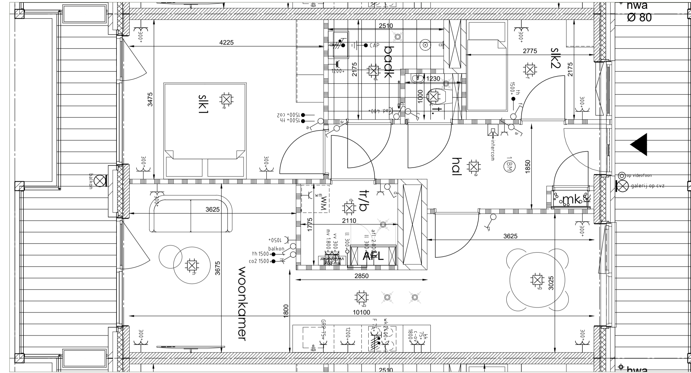
Plattegrond 1:50
