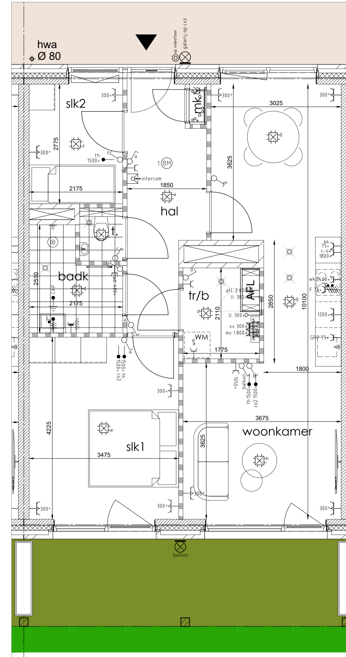
Plattegrond 1:50
