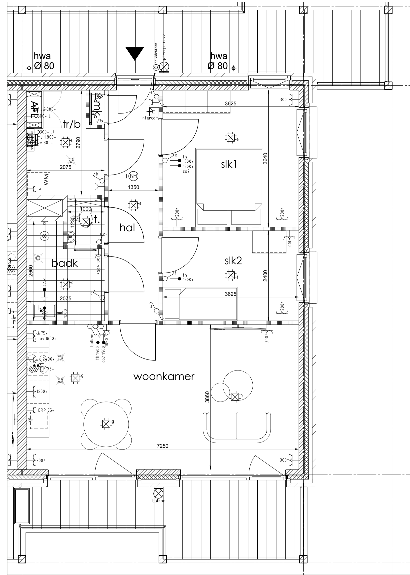
Plattegrond 1:50
