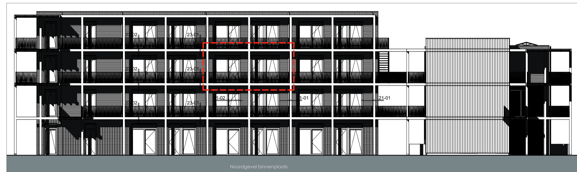
Noordgevel Binnengevel - 1:200
