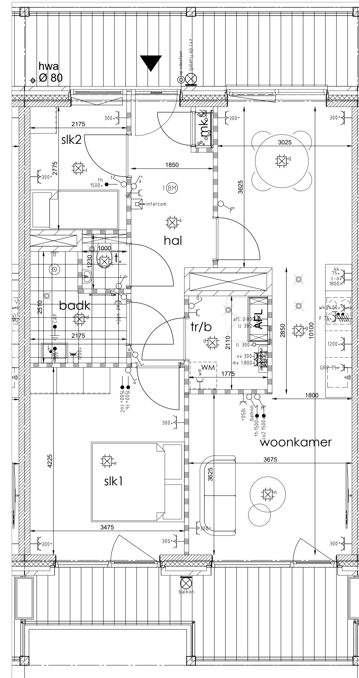
Plattegrond 1:50
