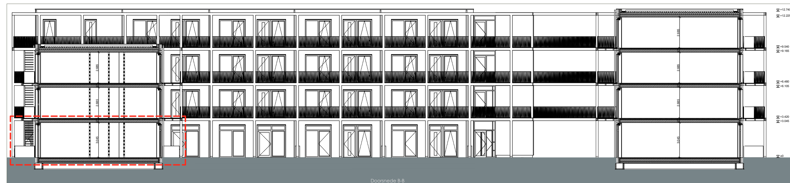
Doorsnede 1:200
