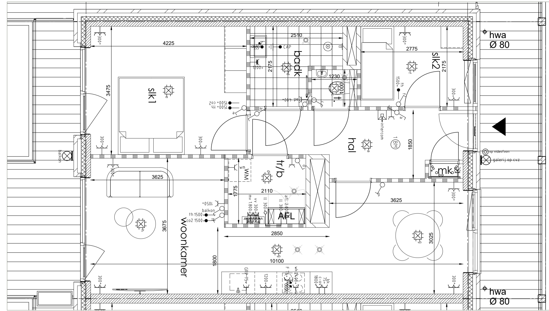
Plattegrond 1:50
