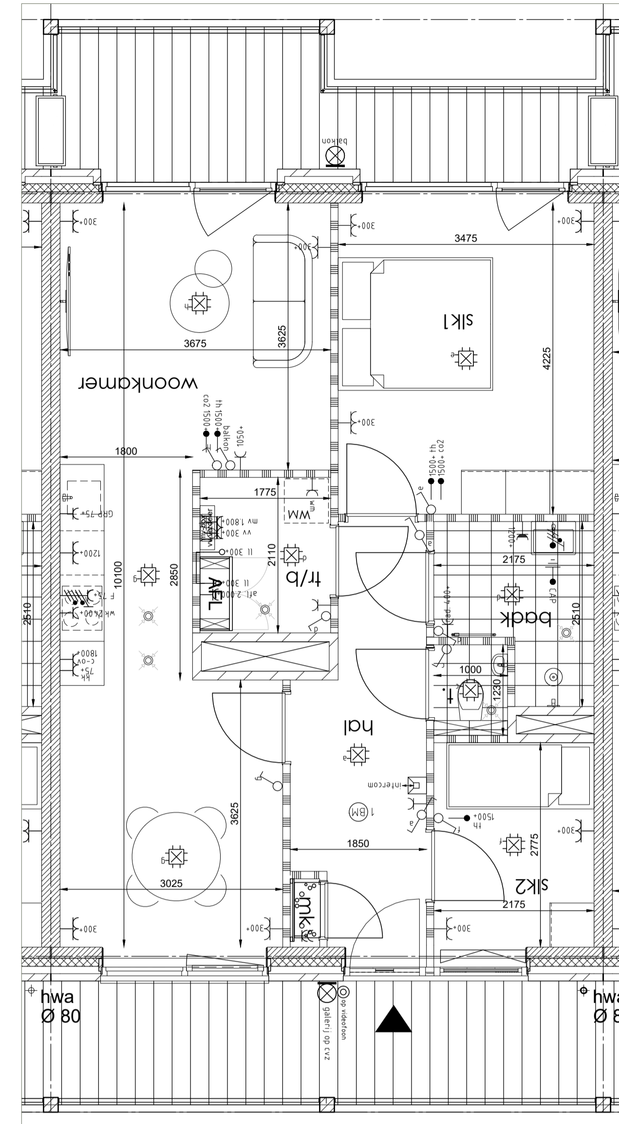
Plattegrond 1:50
