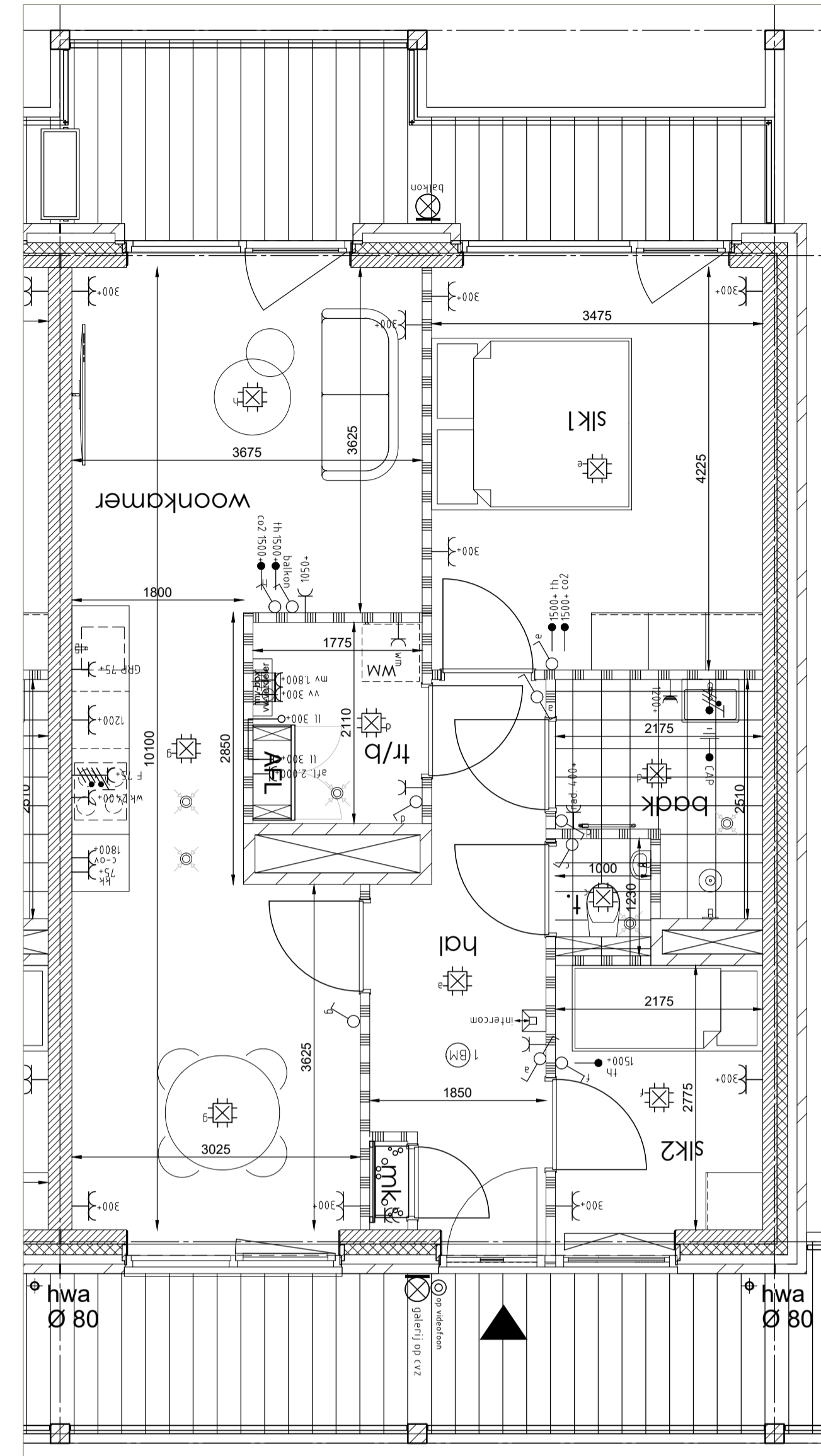
Plattegrond 1:50
