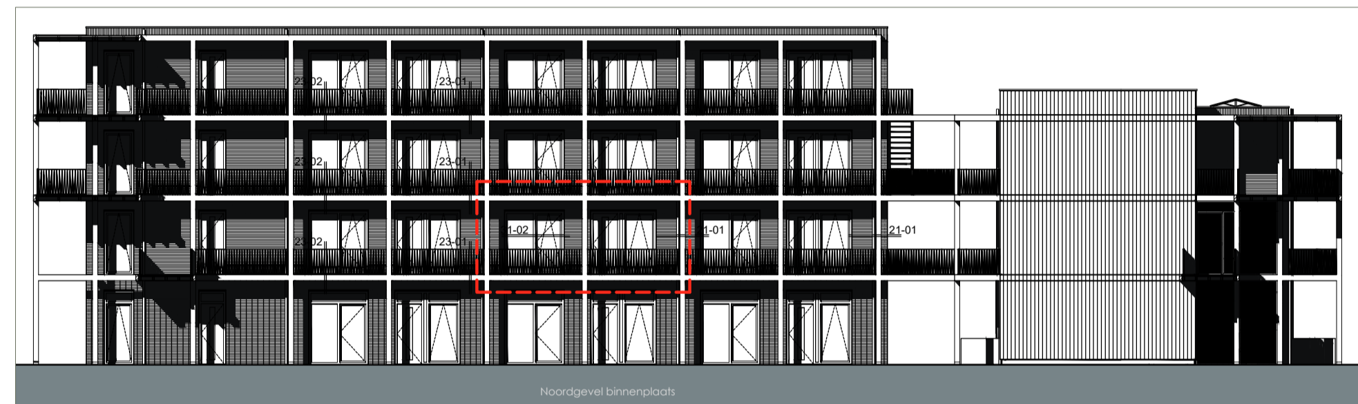
Noordgevel Binnenzijde woonhofje - 1:200
