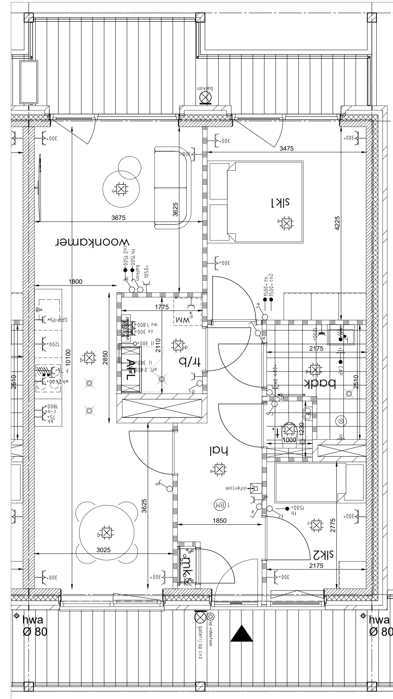
Plattegrond 1:50
