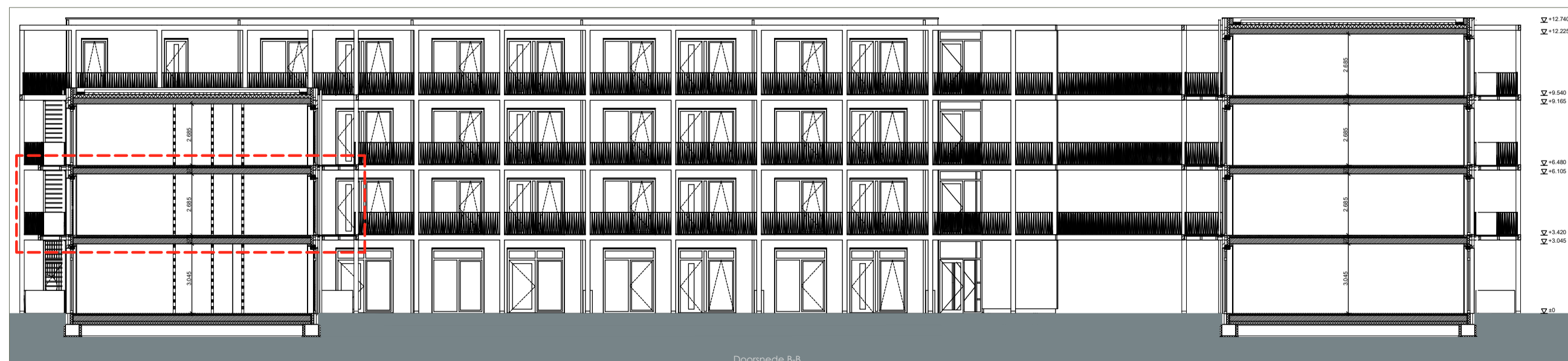
Doorsnede 1:200
