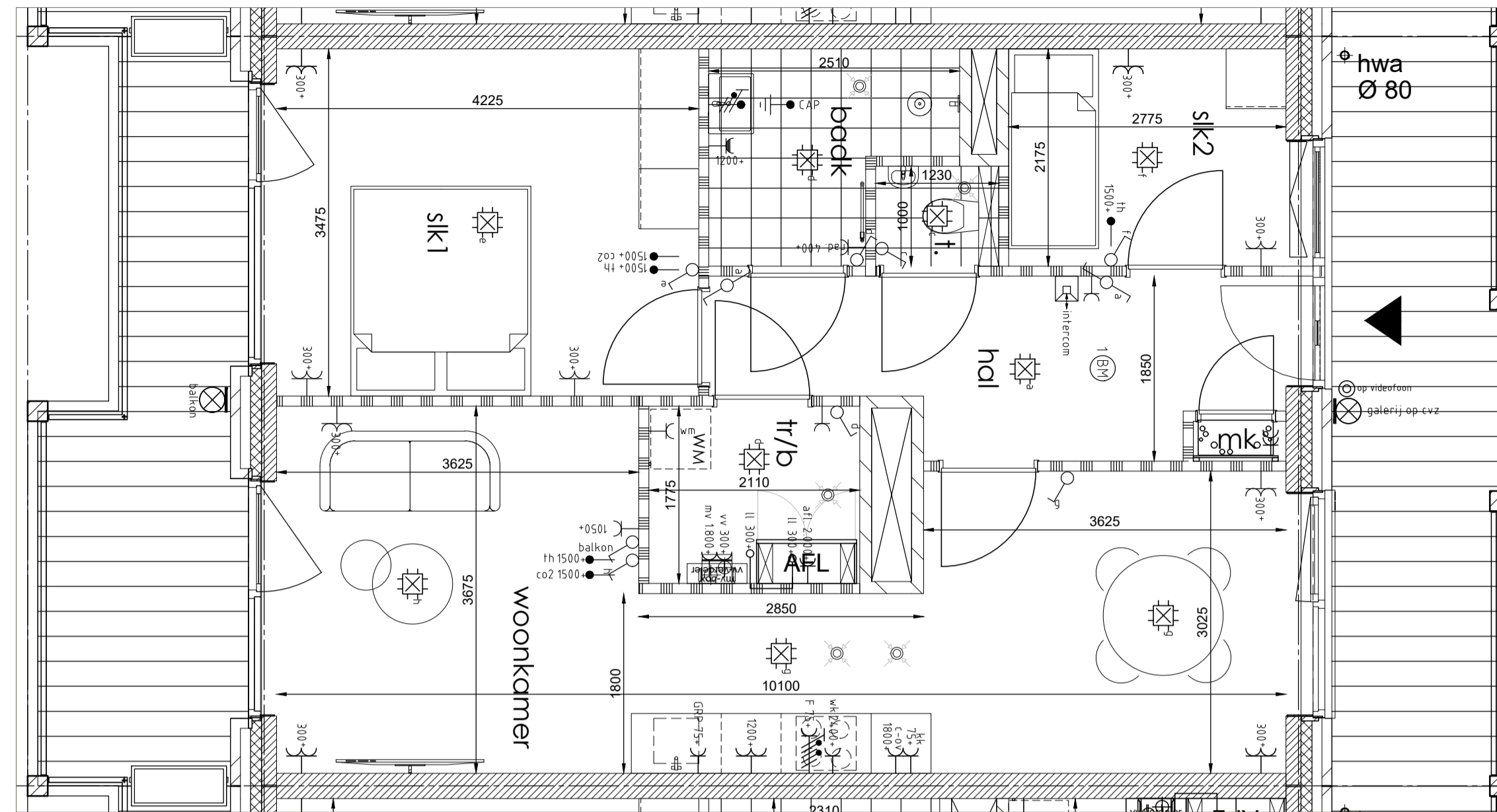
Plattegrond 1:50
