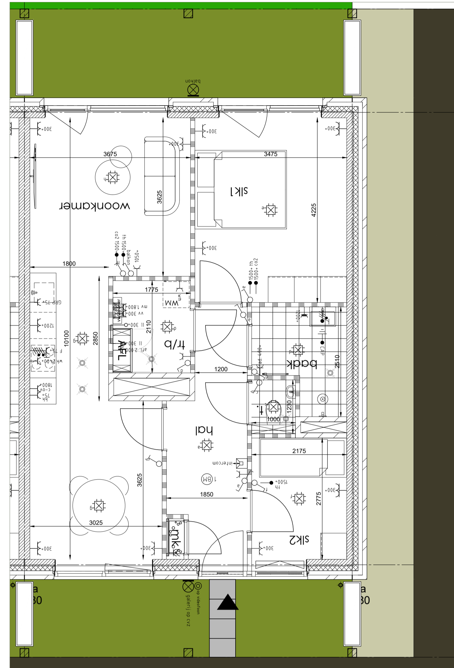
Plattegrond 1:50
