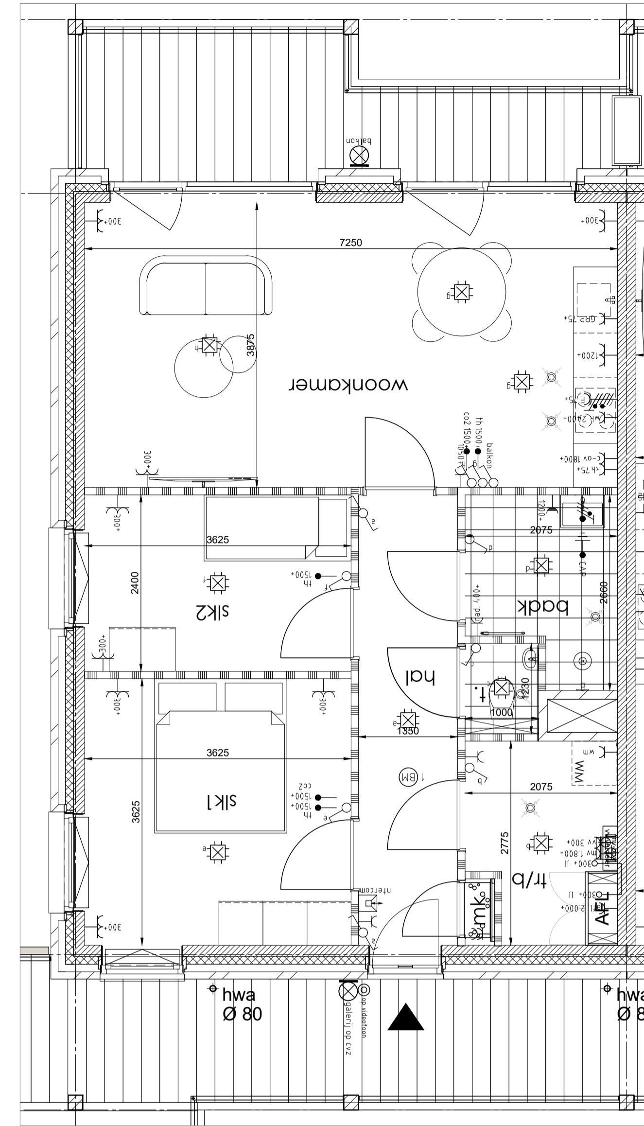
Plattegrond 1:50
