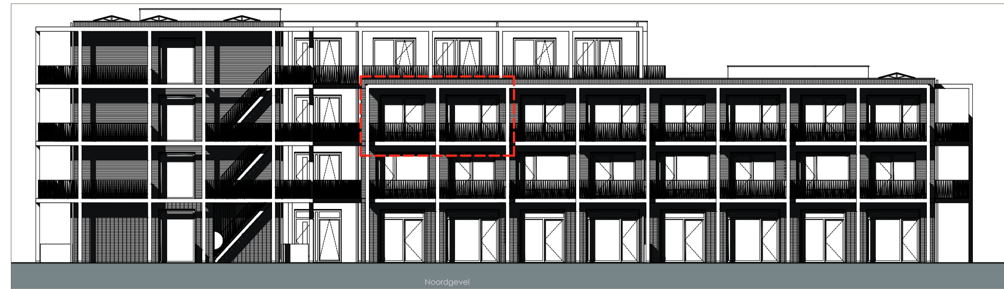
Noordgevel Buitengevel - 1:200
