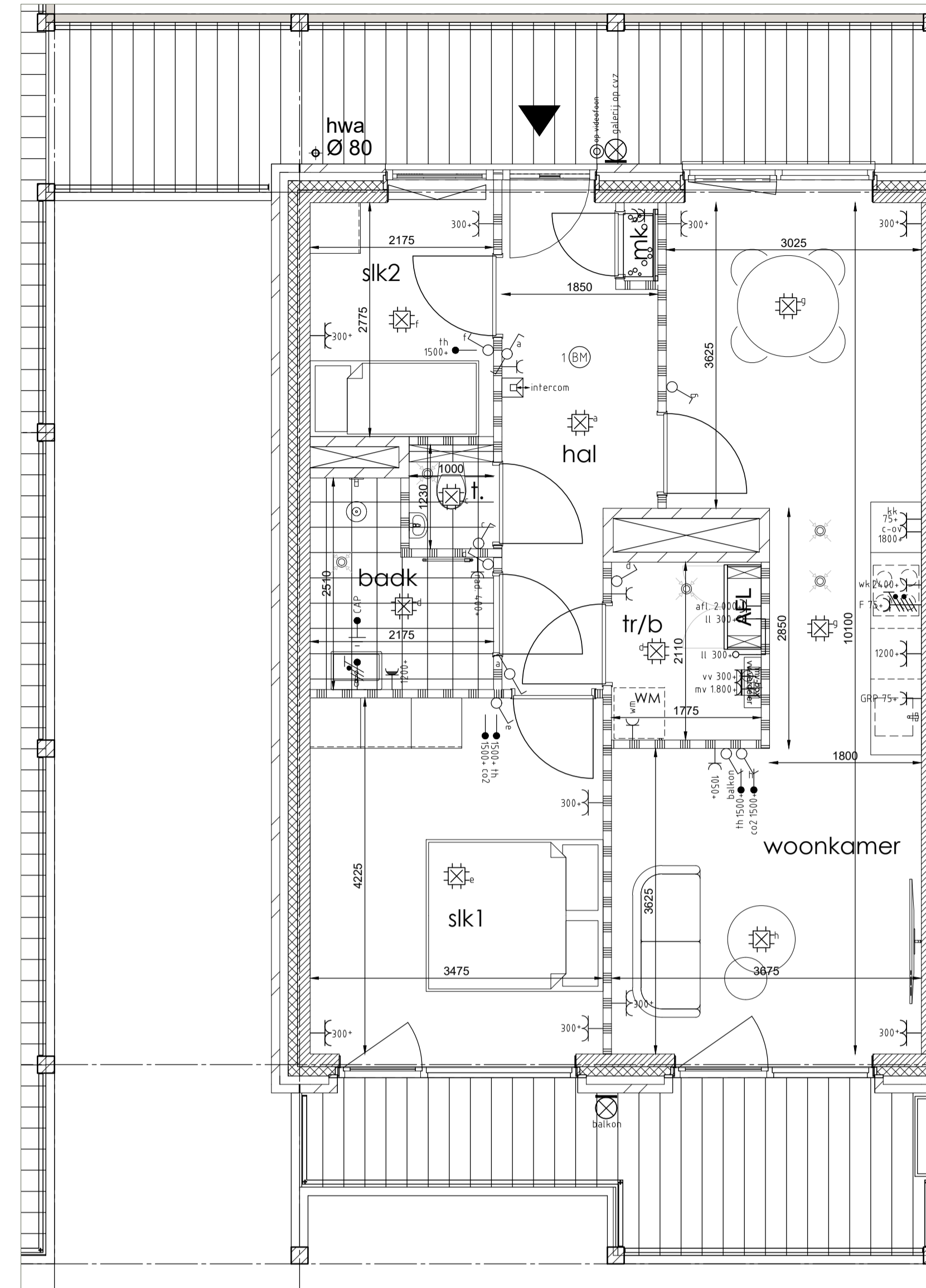
Plattegrond 1:50
