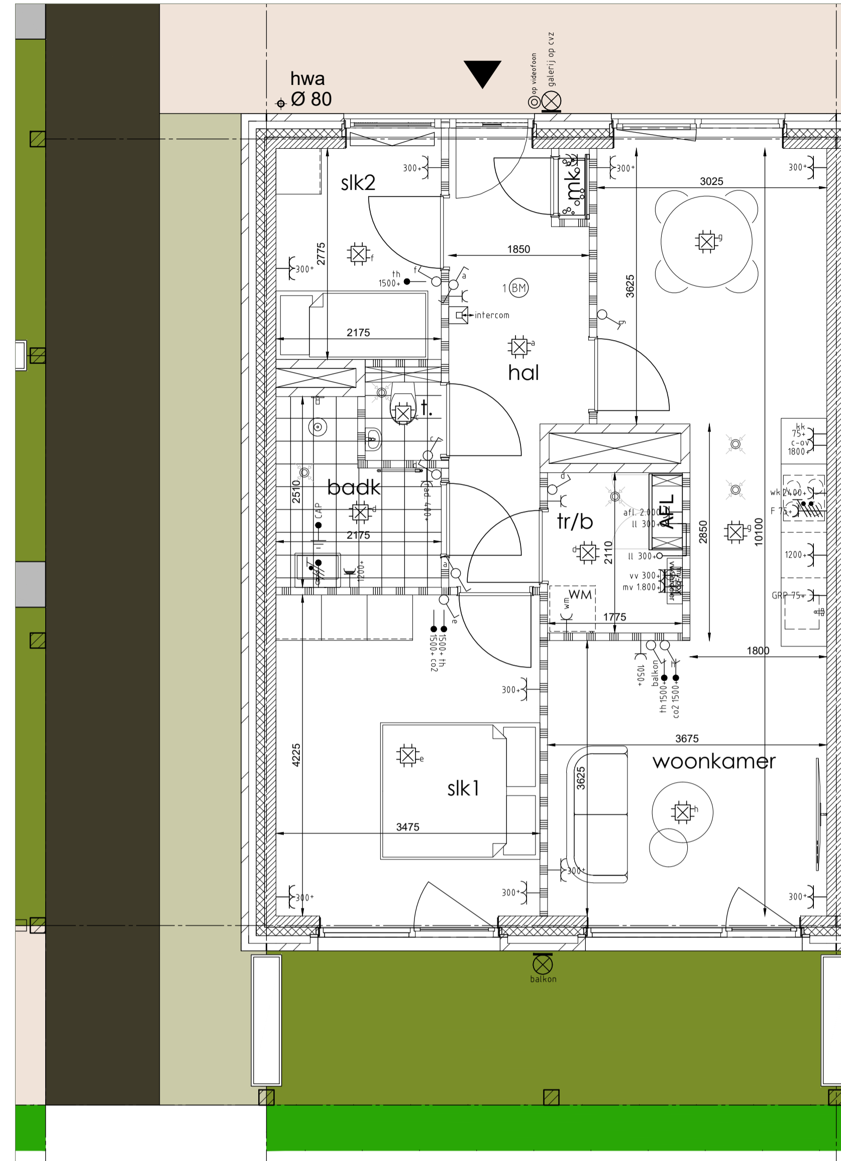
Plattegrond 1:50
