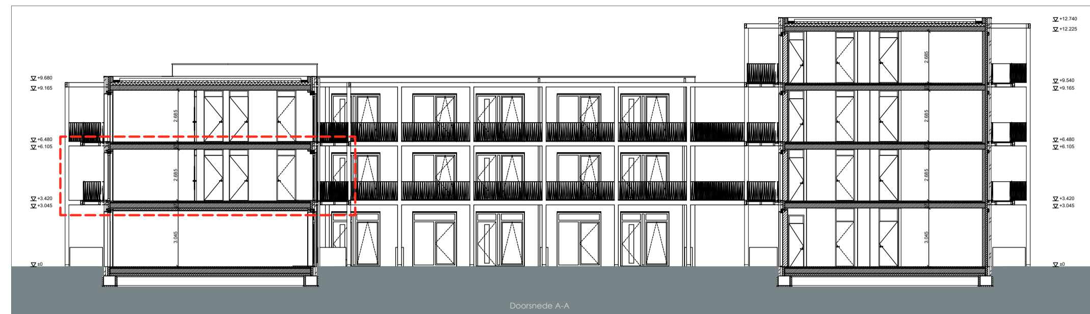
Doorsnede 1:200
