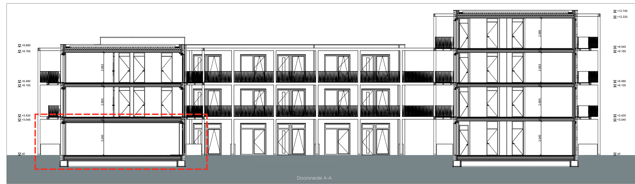
Doorsnede 1:200
