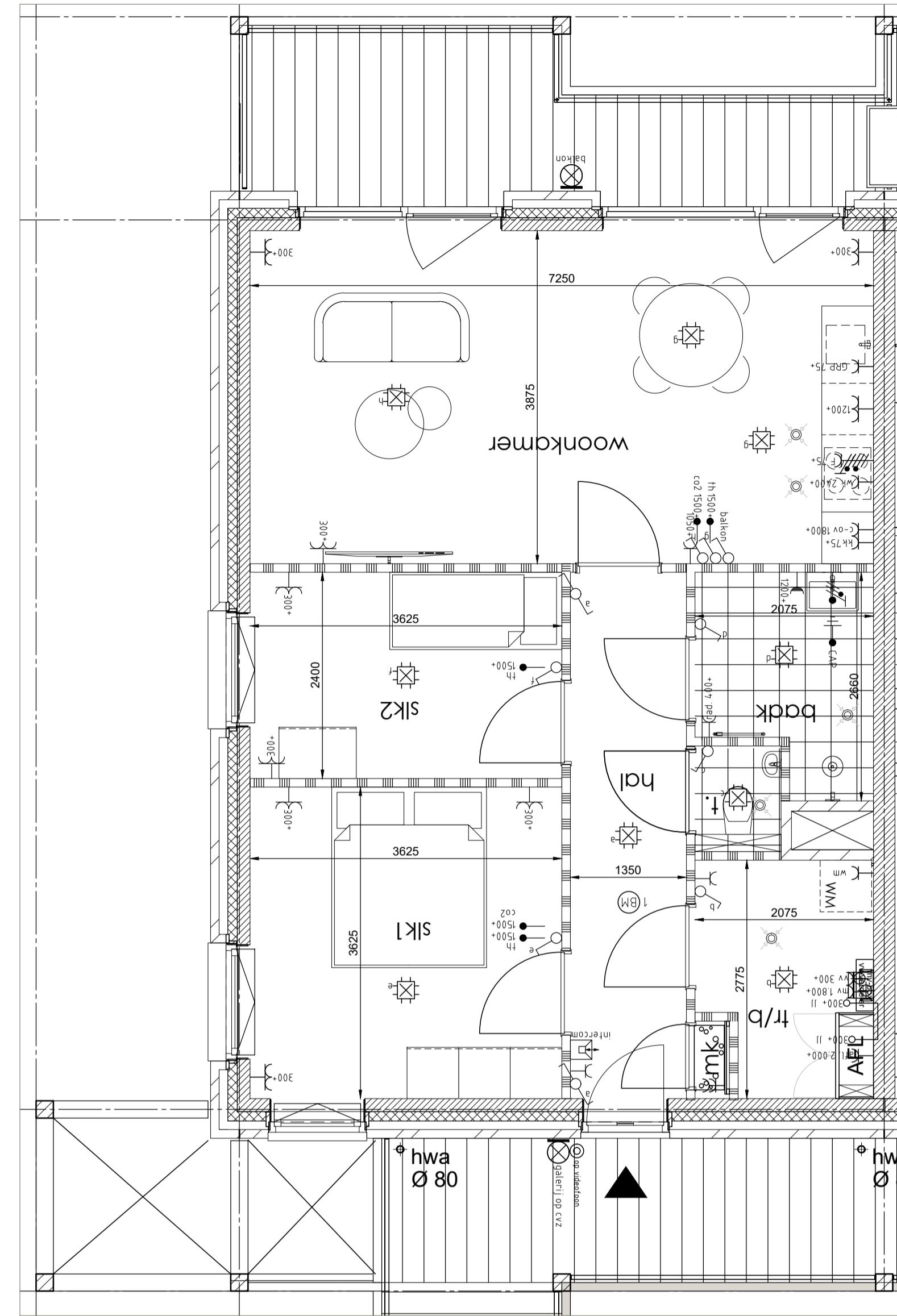
Plattegrond 1:50
