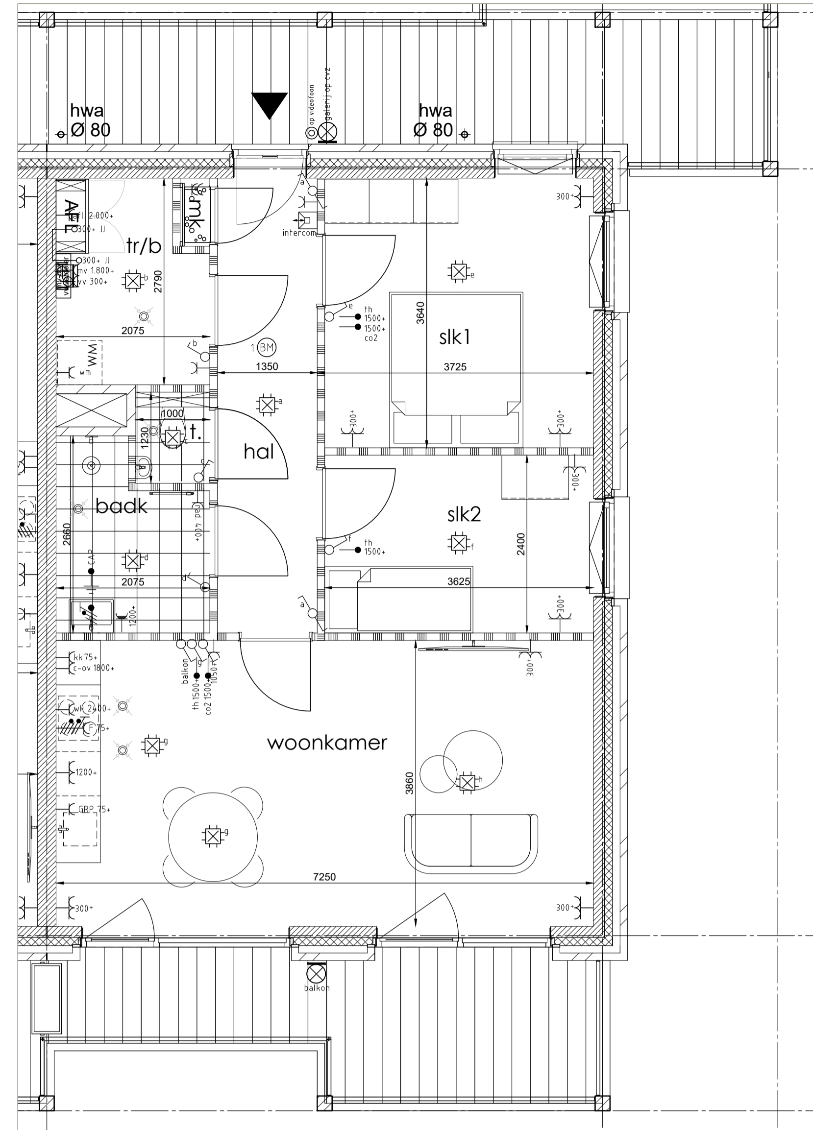
Plattegrond 1:50
