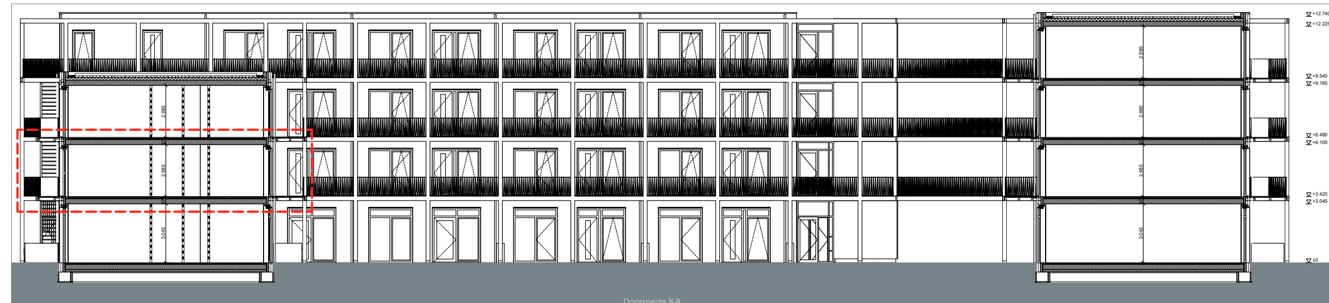
Doorsnede 1:200
