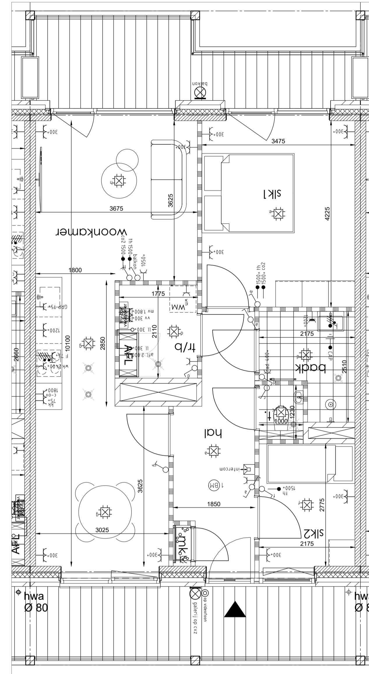
Plattegrond 1:50
