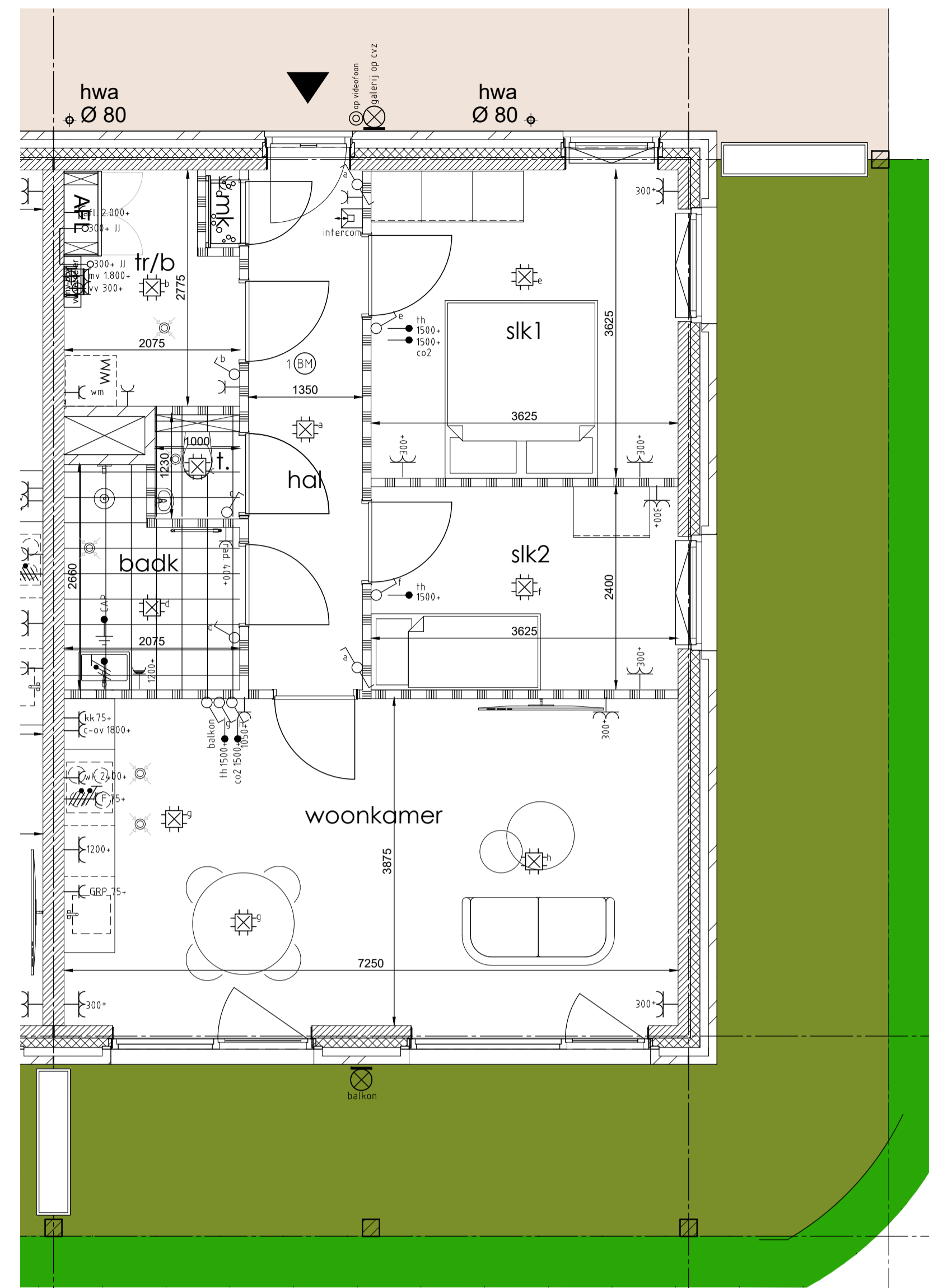
Plattegrond 1:50
