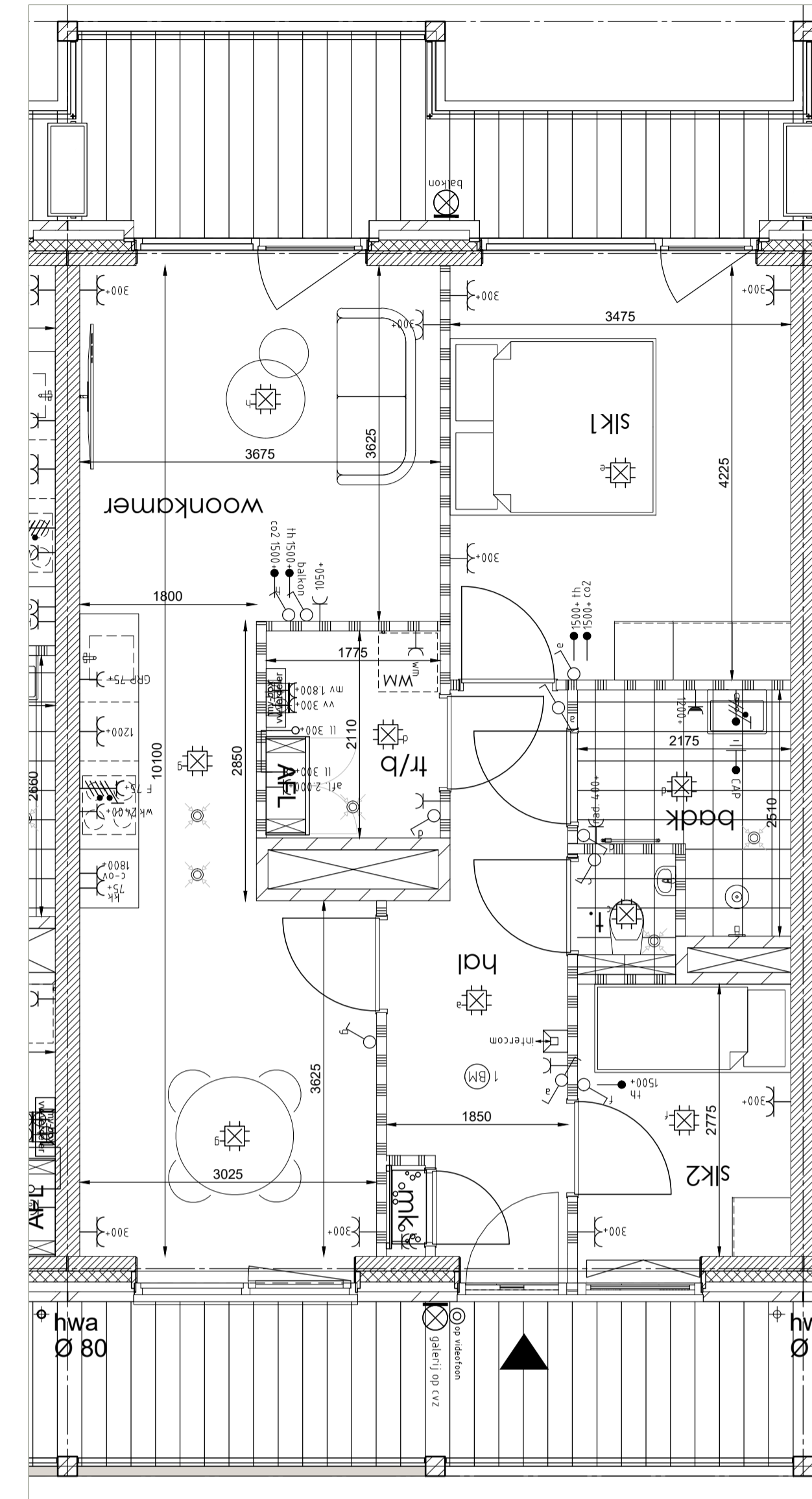
Plattegrond 1:50
