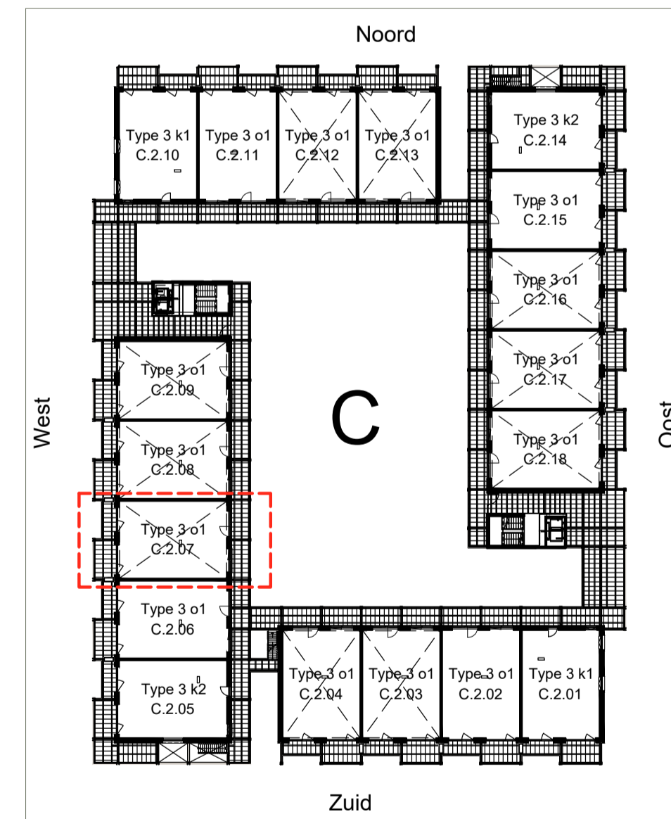
Situatie 1:500 2e Verdieping
