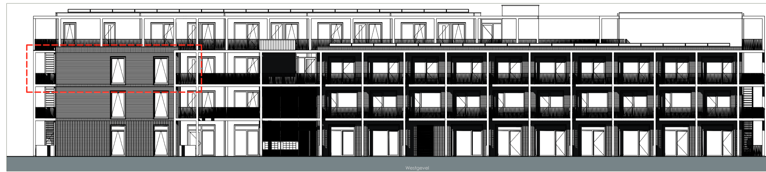
Westgevel Buitengevel - 1:200
