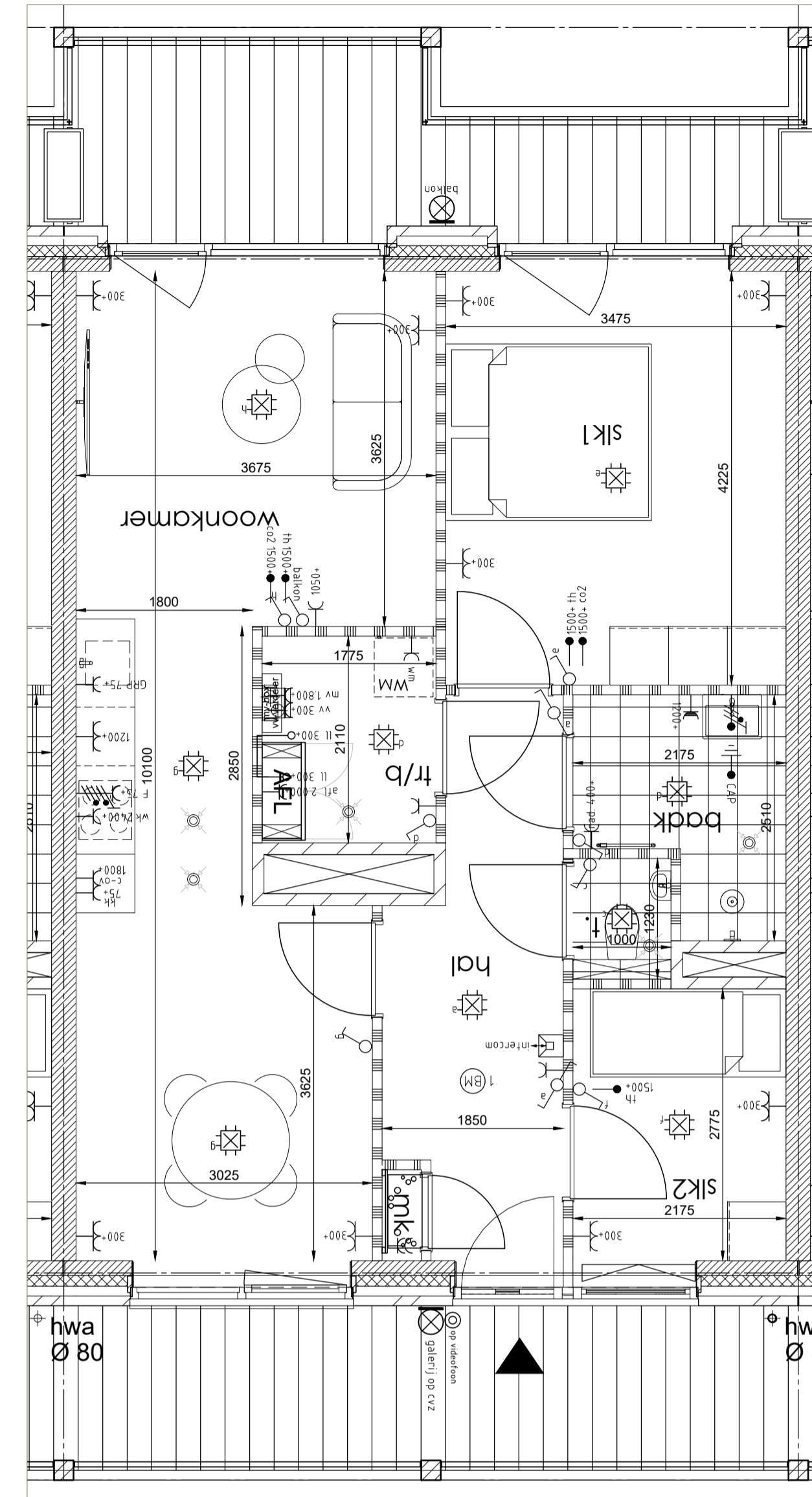
Plattegrond 1:50
