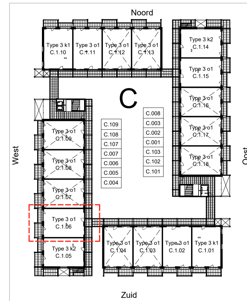
Situatie 1:500 1e Verdieping
