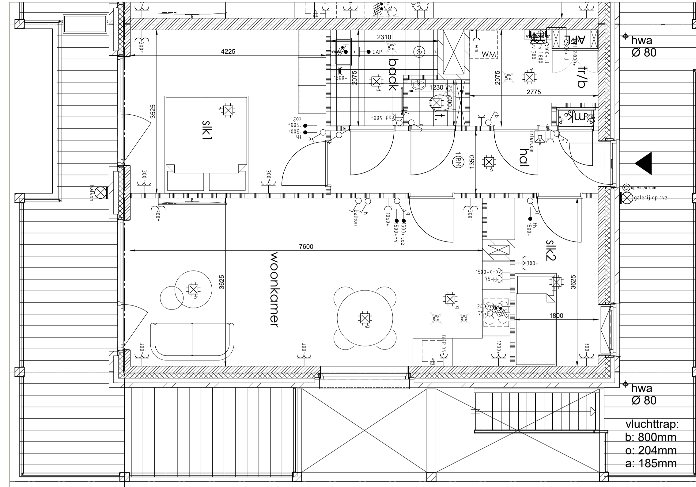
Plattegrond 1:50
