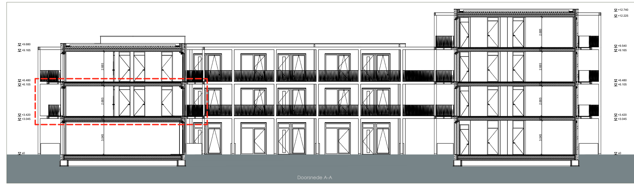
Doorsnede 1:200
