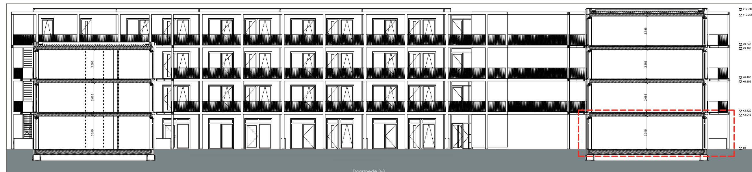
Doorsnede 1:200
