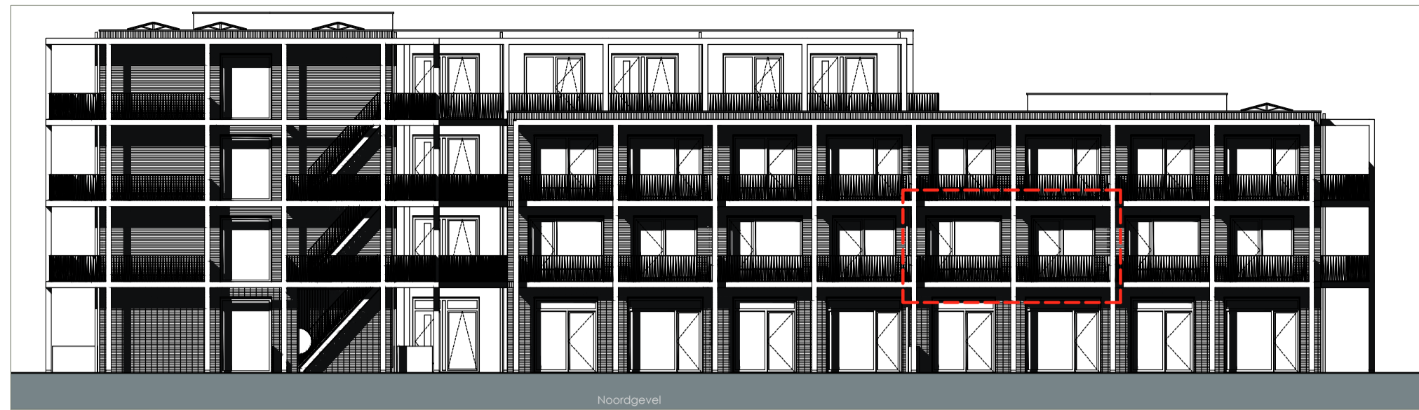
Noordgevel Buitengevel - 1:200
