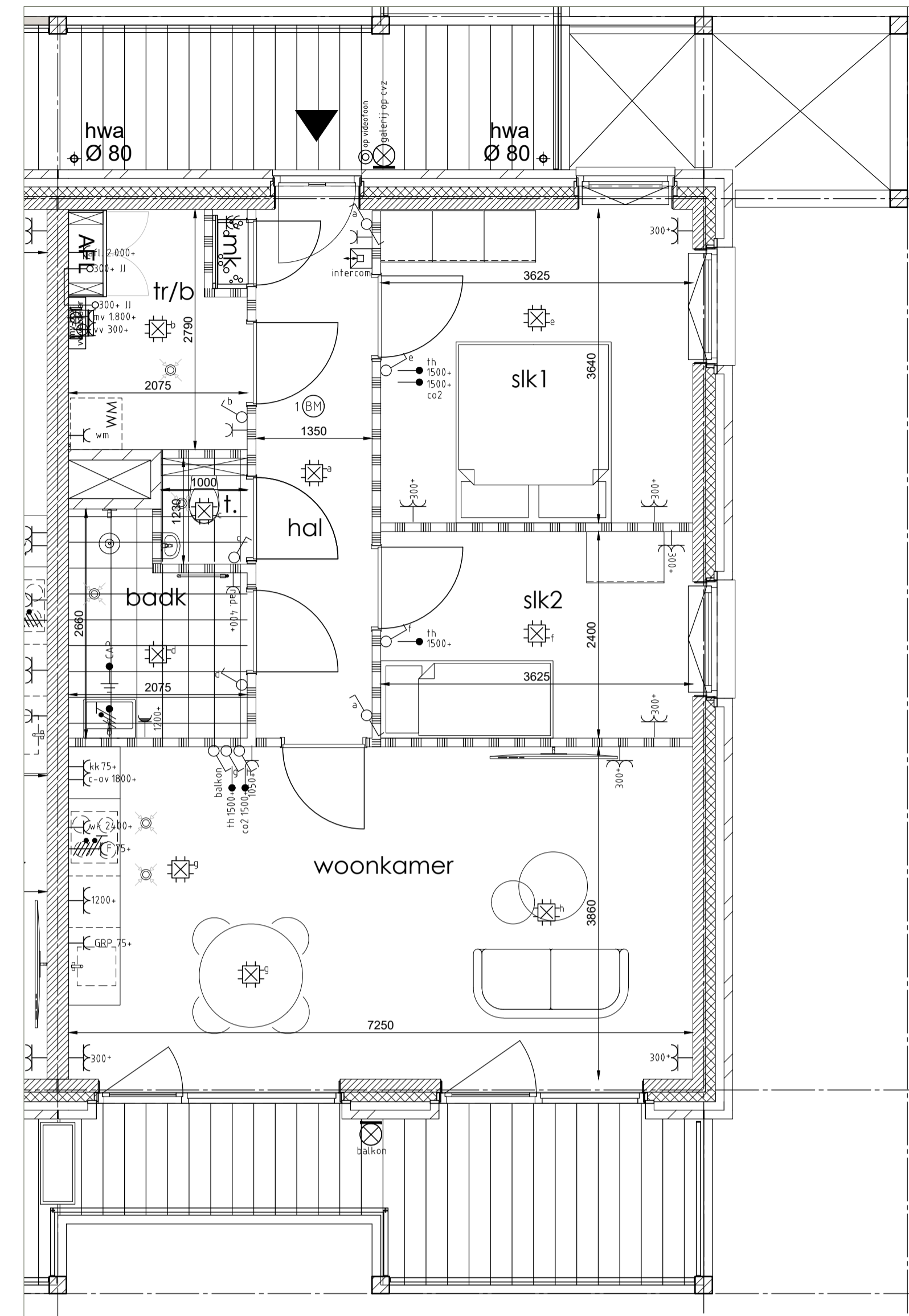
Plattegrond 1:50
