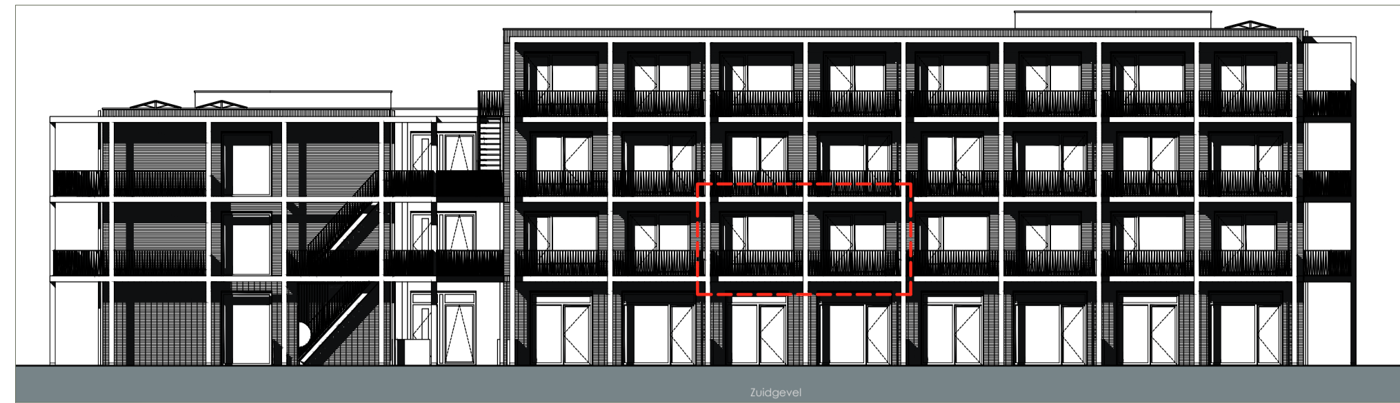
Zuidgevel Buitengevel - 1:200
